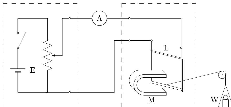
図 8.3: 電磁力を測定する結線図
