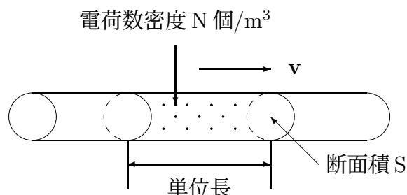
図 8.1: 電荷の移動
