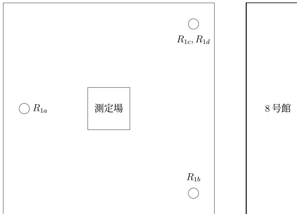
図 10.2: 接地抵抗の測定場所
