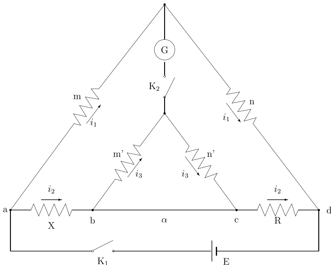
図 8.1: ダブルブリッジの原理図
