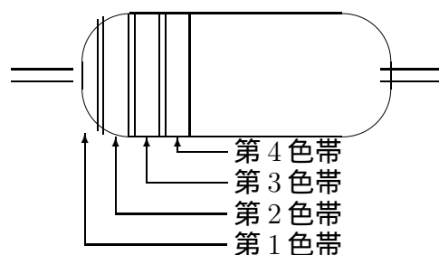
図 1.2: 固定抵抗器のカラーコード
