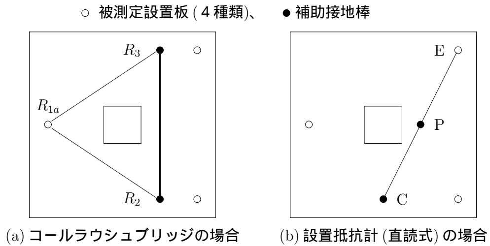
図 11.2: 接地抵抗の測定場所
