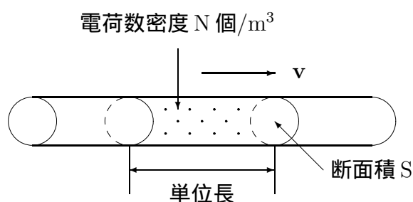
図 19.1: 電荷の移動
