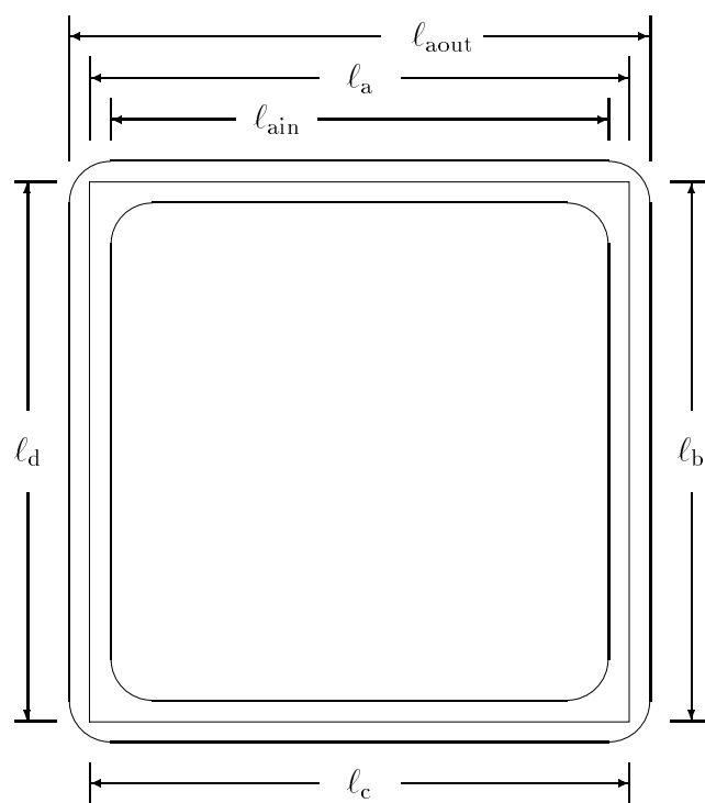
図 19.5: コイル導線の長さの測定
