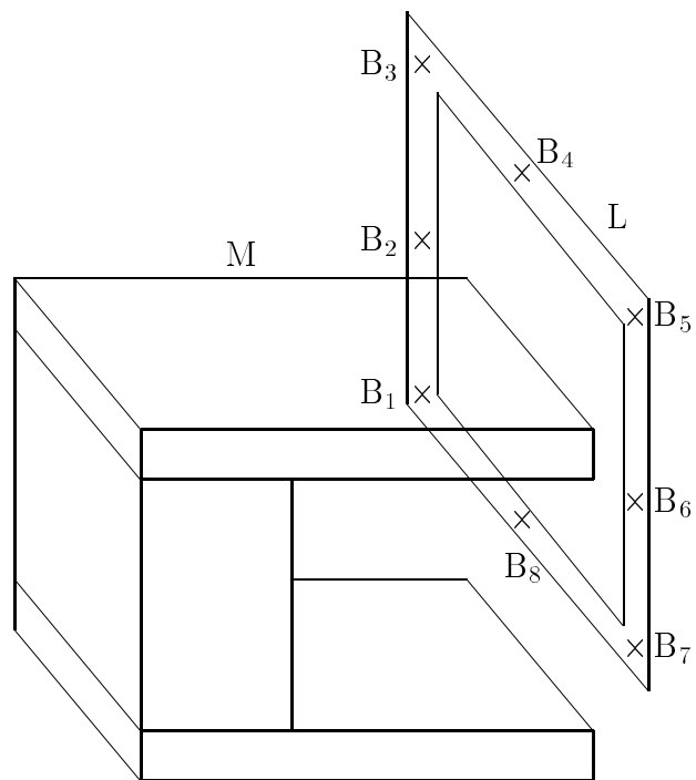
図 19.4: 磁束密度の測定
