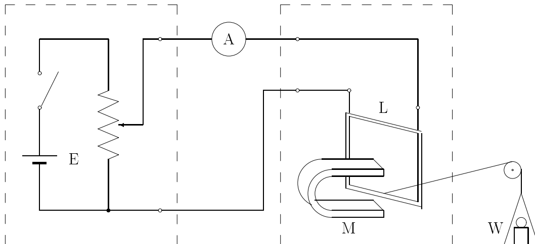
図 17.3: 電磁力を測定する結線図
