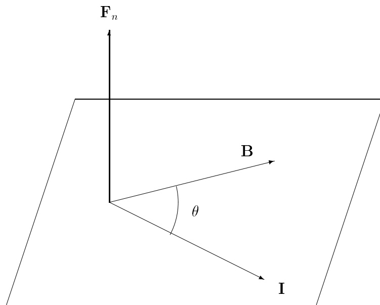
図 17.2: 磁界中の電流に働く力のベクトル図
